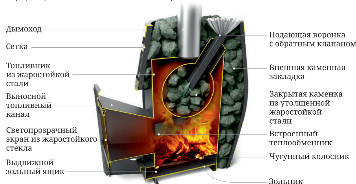
На разрезе представлена печь «Саяны XXL 2015 Витра»
